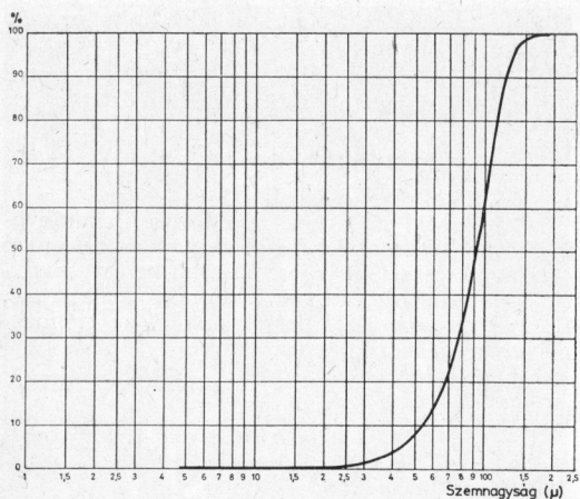
12. ábra. Kitöltés anyagának szemeloszlási görbéje
