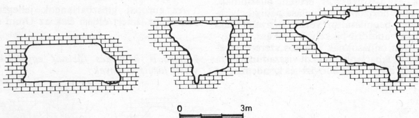
9. ábra. Sík főtek három jellegzetes szakasz szelvényében
