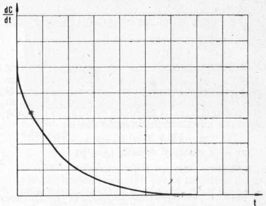
1. ábra. A gipsz oldódása
