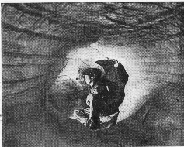
5. ábra. Csőszerű, inaktív járat
