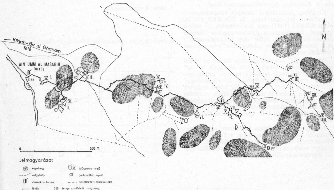
4. ábra. A barlangrendszer alaprajza és felszíni kapcsolatai
