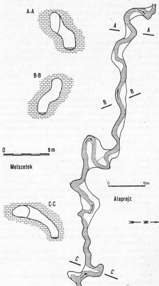
17. ábra. Meanderező járatszakasz alaprajza és metszetei
