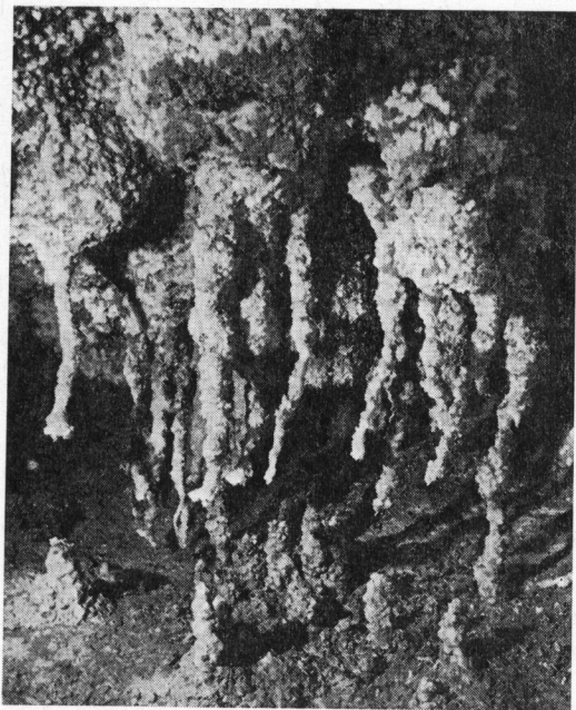
18. ábra. Gipsz-cseppkövek
